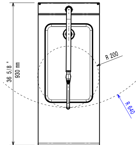
Boven aanzicht
